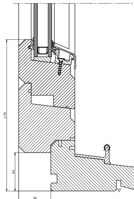
Tegning nr. 4-47-28, vertikalt snitt. Vi sender gjerne illustrasjoner i DWG- eller DXF-format, på forespørsel. Disse viser vertikale og horisontale snitt, vinduspostene og alternative glasstyper.
