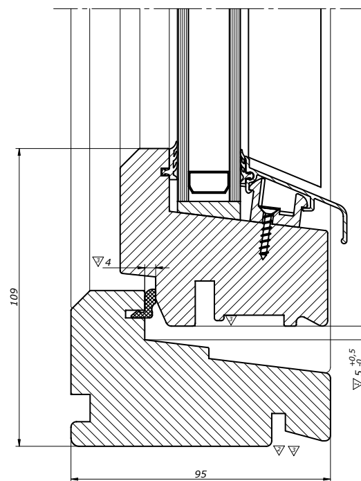
Tegning nr. 4-44-07, vertikalt snitt. Vi sender gjerne illustrasjoner i DWG- eller DXF-format, på forespørsel. Disse viser vertikale og horisontale snitt, vinduspostene og alternative glasstyper.
