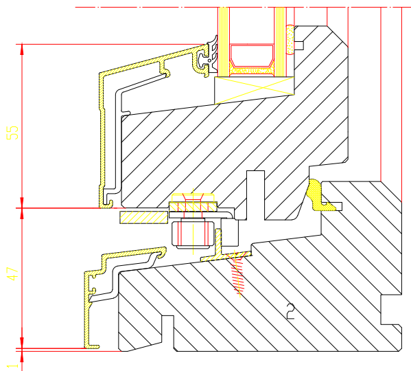
Tegning nr. HSS 2L, vertikalt snitt. - bekledd med aluminium.
