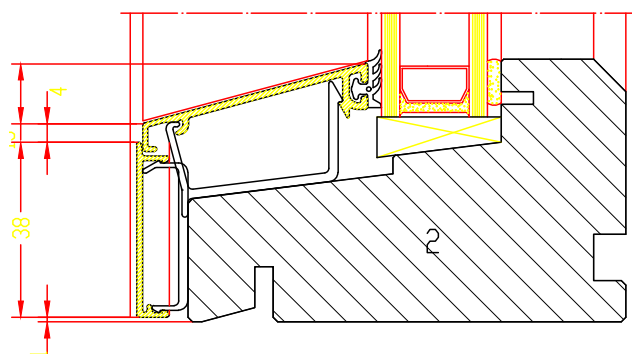
Tegning nr. HFK 2L, vertikalt snitt. - bekledd med aluminium.
