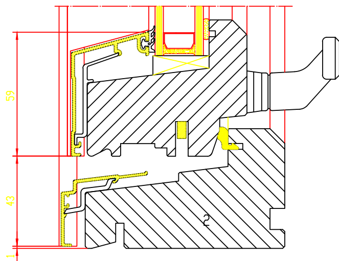
Tegning nr. HTS 2L, vertikalt snitt - bekledd med aluminium.
