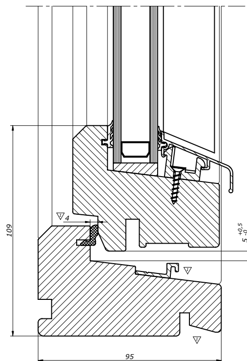
Tegning nr. 4-45-86 vertikalt snitt. Vi sender gjerne illustrasjoner i DWG- eller DXF-format, på forespørsel. Disse viser vertikale og horisontale snitt, vinduspostene og alternative glasstyper.
