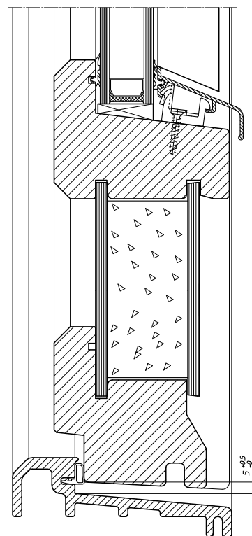
Tegning nr. 4-45-80 vertikalt snitt. Vi sender gjerne illustrasjoner i DWG- eller DXF-format, på forespørsel. Disse viser vertikale og horisontale snitt, vinduspostene og alternative glasstyper.
