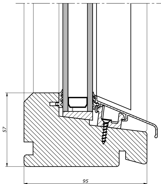
Tegning nr. 4-44-23, vertikalt snitt. Vi sender gjerne illustrasjoner i DWG- eller DXF-format, på forespørsel. Disse viser vertikale og horisontale snitt, vinduspostene og alternative glasstyper.
