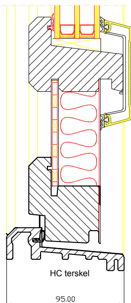
Tegning nr. HB ALU HC, vertikalt snitt. - bekledd med aluminium.
