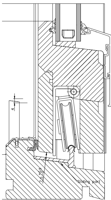
Tegning nr. 4-47-31 vertikalt snitt. - bekledd med aluminium.
